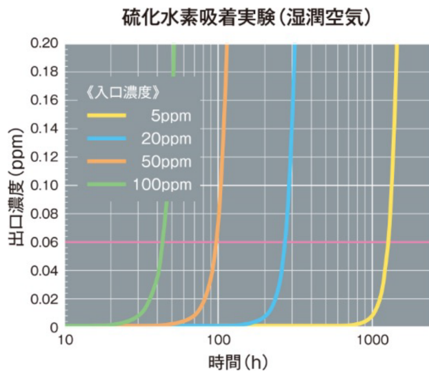
真空ポンプの排気対策による効果予測
